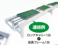
苗送りローラー NR-18 24,000円
